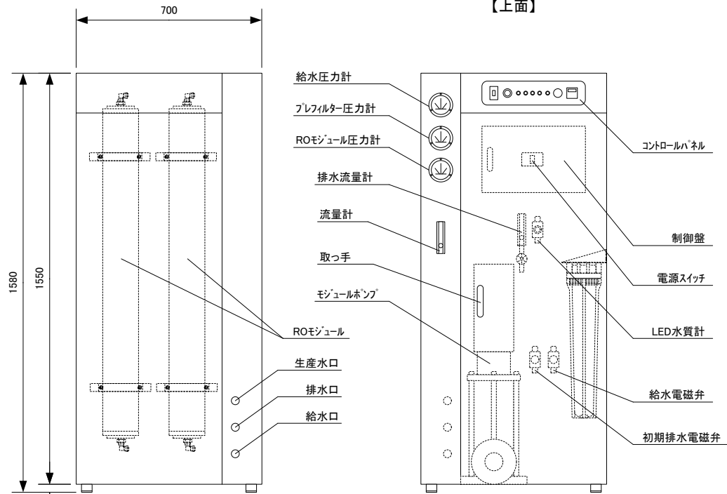
【正面】
