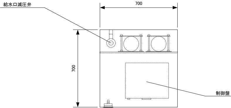
【上面】
