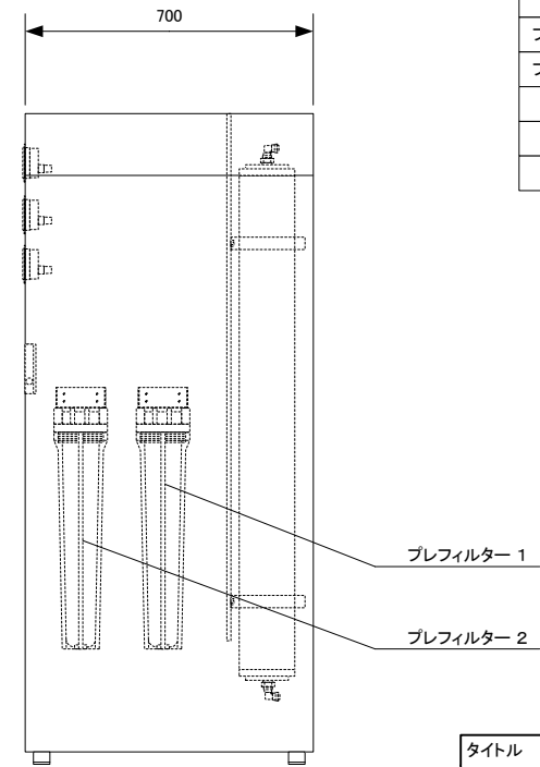
【側面】
